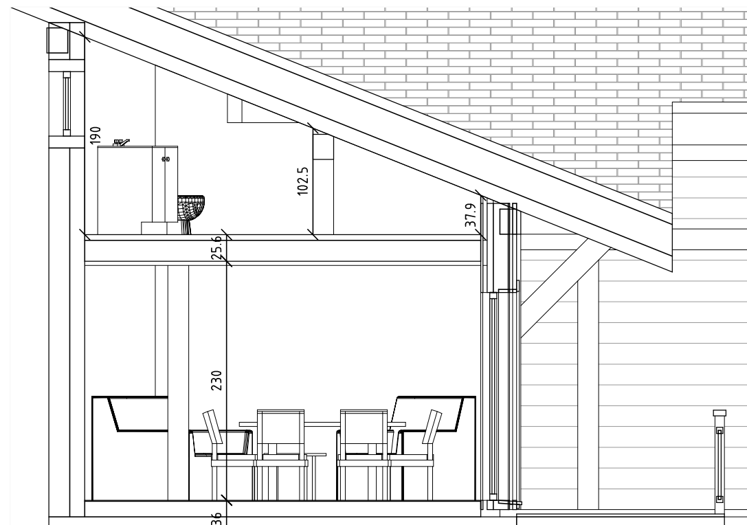
Coupe 1er Etage & Mezzanine
